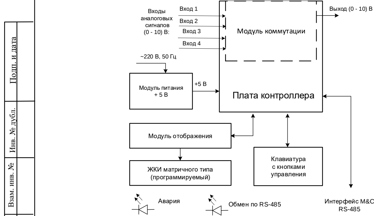
Рисунок 1.2 - Функциональная схема АК 1х4
